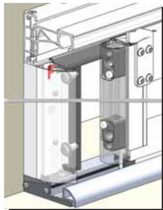
2 points de verrouillage côté fermeture (1 point bas et 1 point haut).
