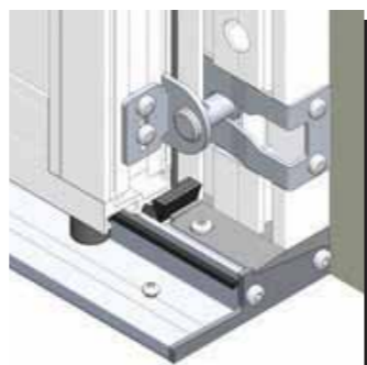
1 point de verrouillage côté refoulement (1 point bas).
