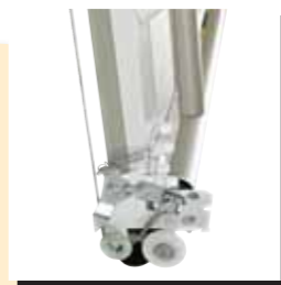
Parachute câble sécurité "Stop chute".
